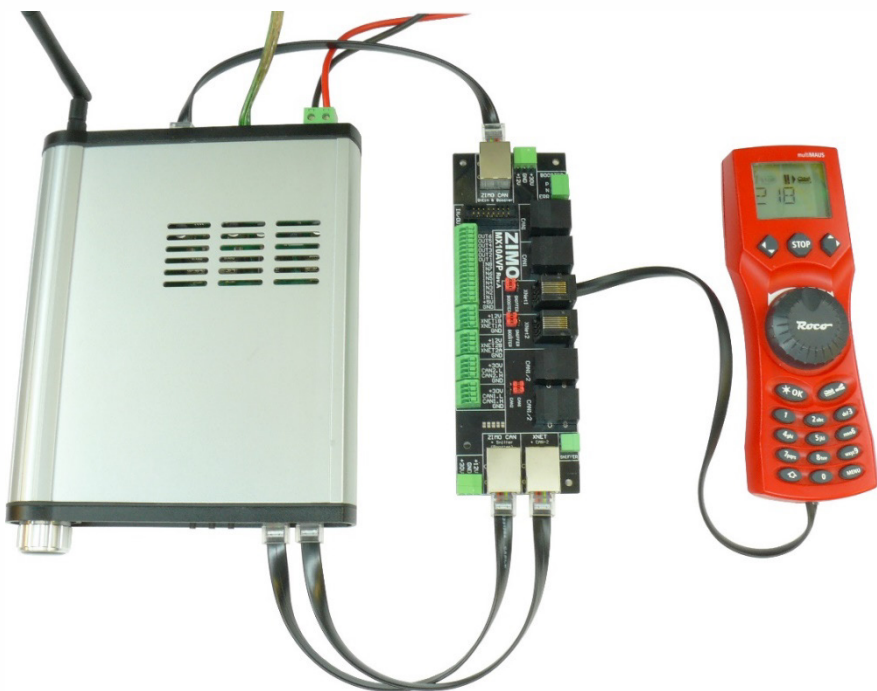
Anschluss einer Roco multiMÄUSE über ein 6-poliges Kabel an einer XNET Buchse der MX10AVP (natürlich wäre zum Anschluss einer einzigen multiMÄUSE keine „Anschluss- und Erweiterungsplatine“ notwendig, aber in Kombination mit einem der vorgenannten Fälle ist diese Art des Anschlusses sinnvoll).
